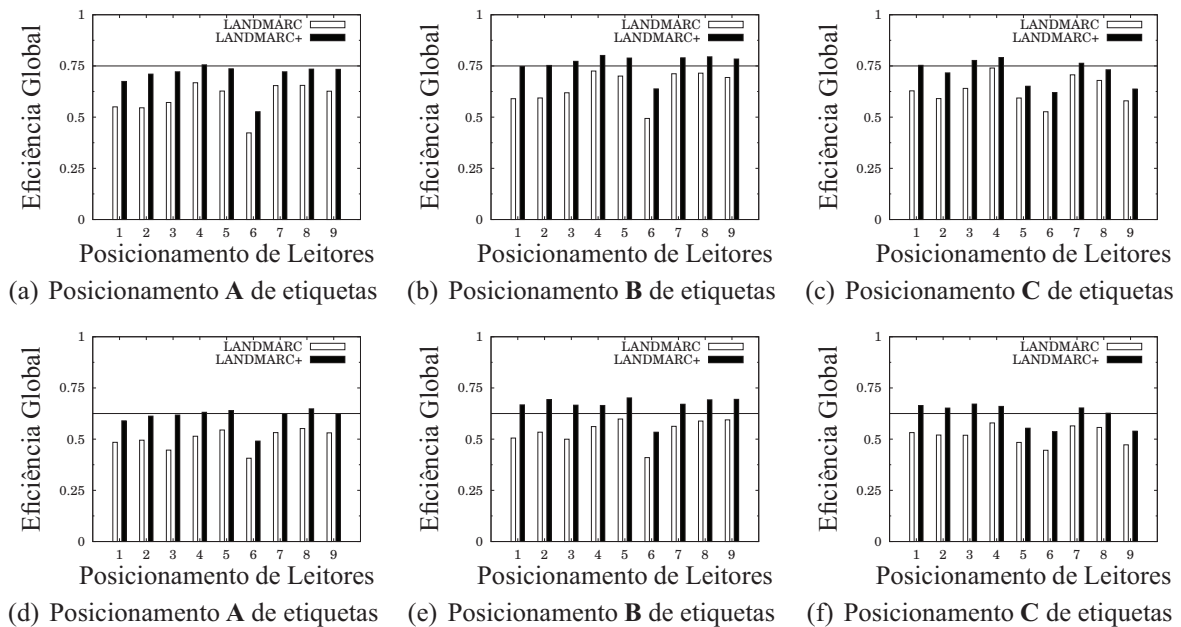
Figura 3. (a), (b) e (c): Cenário 3 (fechado/ Path Loss estendido). (d), (e) e (f): Cenário 4 (aberto/ Path Loss estendido).
