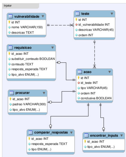
Figura 5. Modelagem Relacional do Banco de Dados da J-Attack
