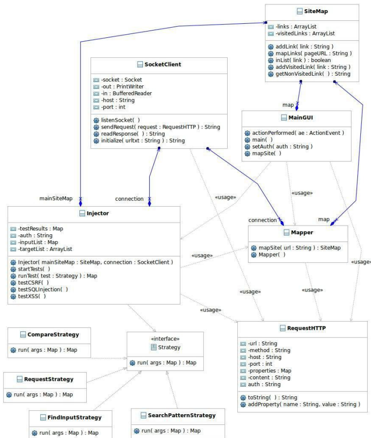
Figura 6. Diagrama de Classes da J-Attack
