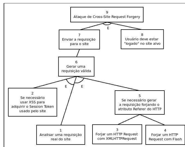
Figura 3. Árvore de Ataque - Cross Site Request Forgery
