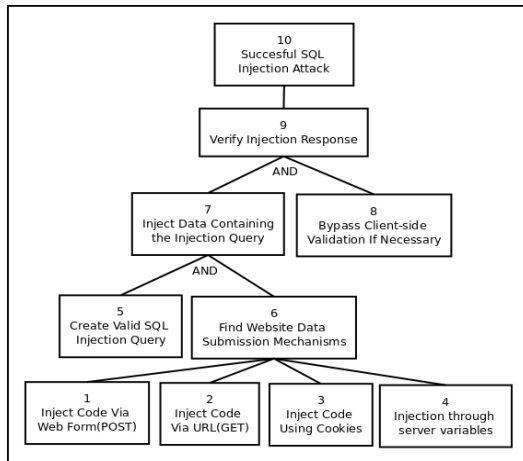
Figura 1. Árvore de Ataque - SQL Injection
