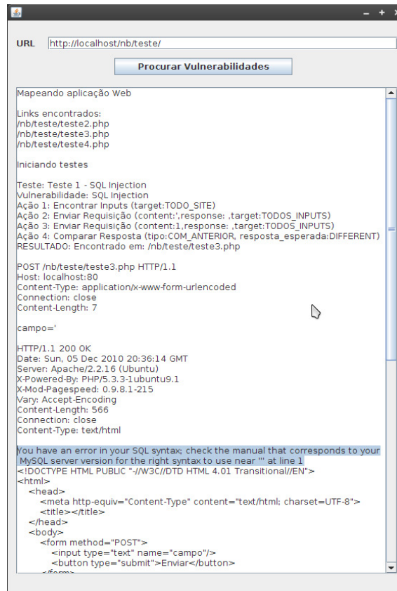
Figura 10. Interface da J-Attack – Execução de ataque SQL Injection
