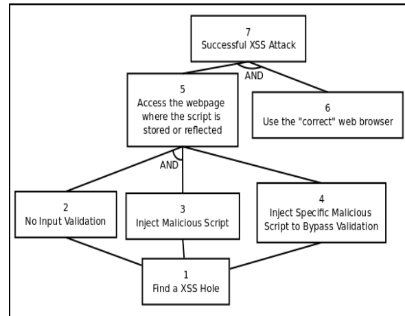
Figura 2. Árvore de Ataque - Cross Site Scripting
